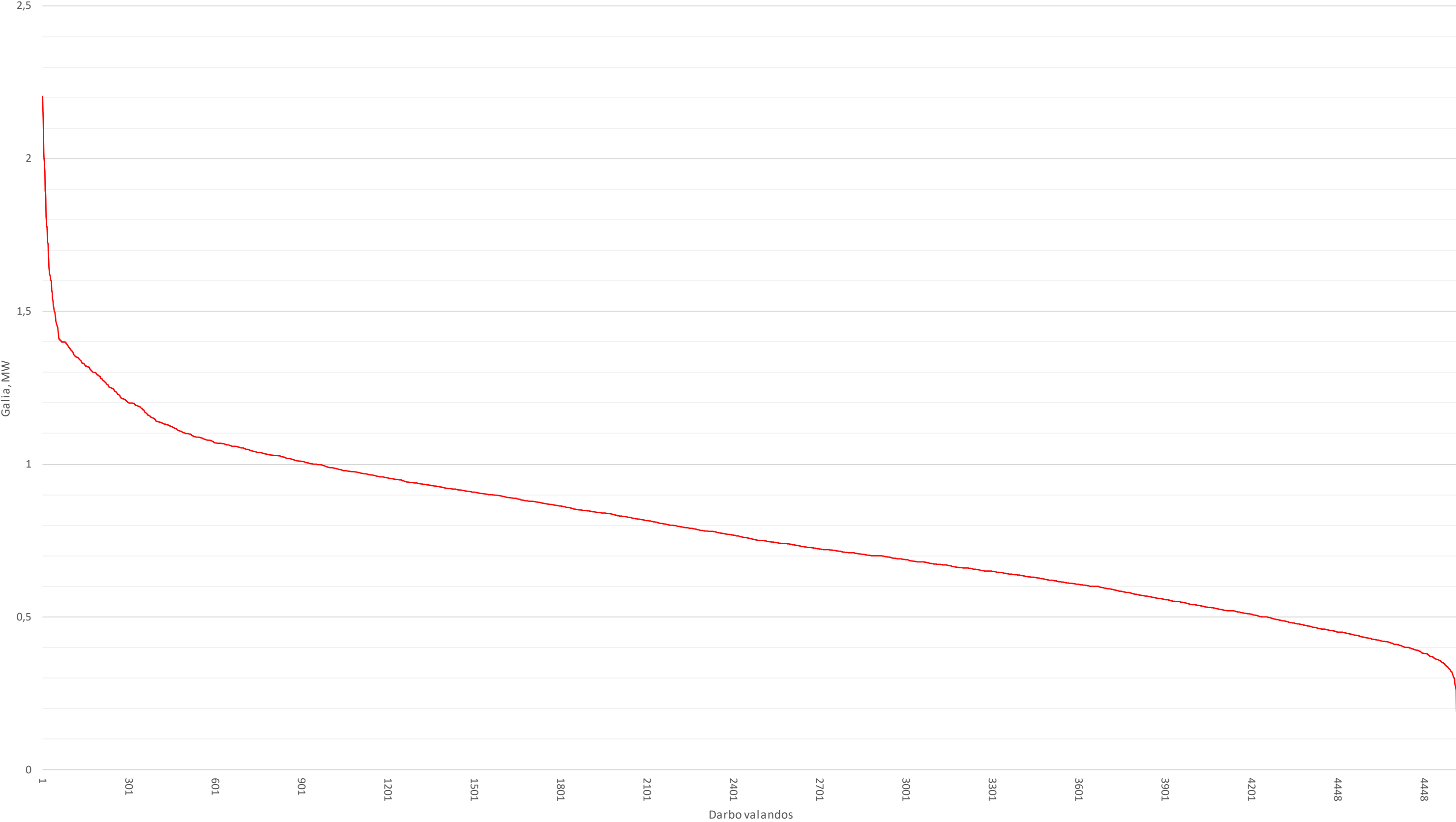
Viešnių katilinės 2024 metų apkrovimo grafikas
