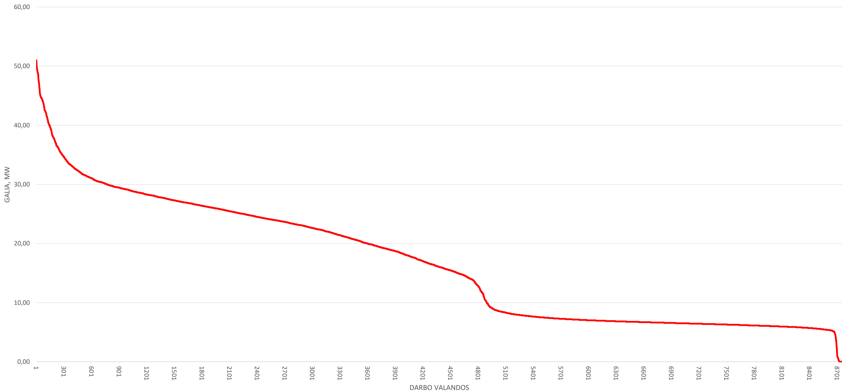
Mažeikių katilinės 2024 metų apkrovimo grafikas
